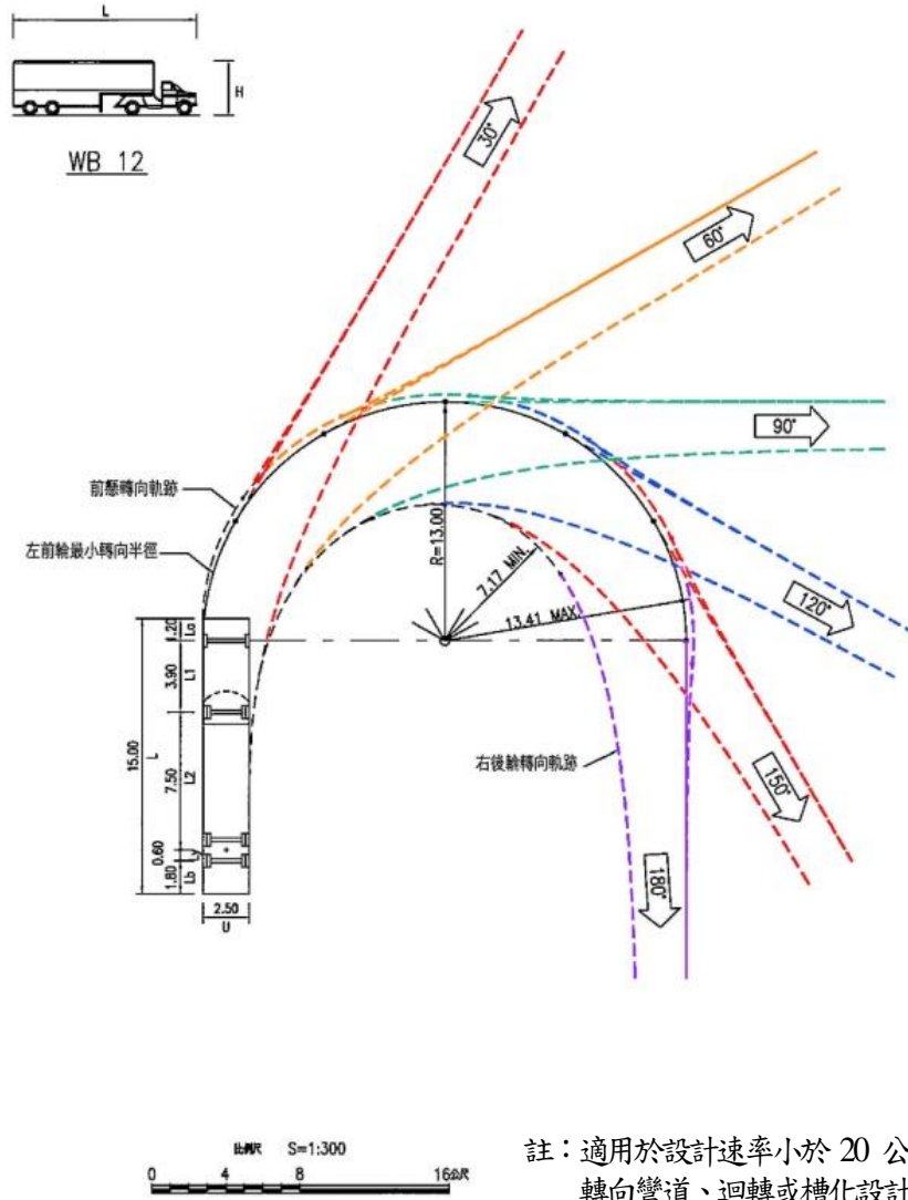
中型聯結車最小轉向軌跡參考圖
