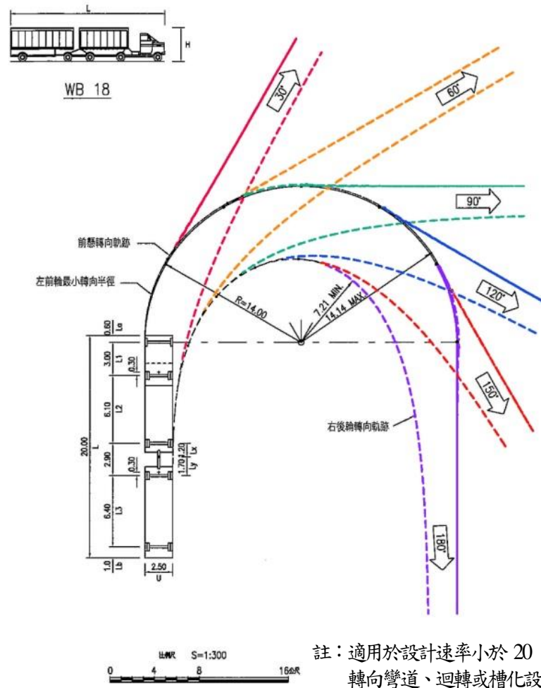
全聯結車最小轉向軌跡參考圖
