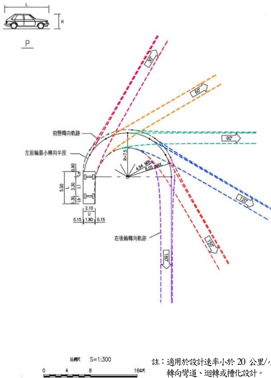
小客車最小轉向軌跡參考圖
