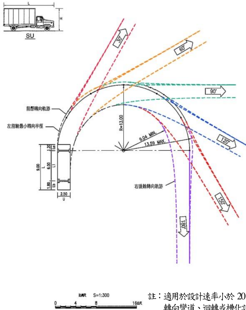
貨車最小轉向軌跡參考圖
