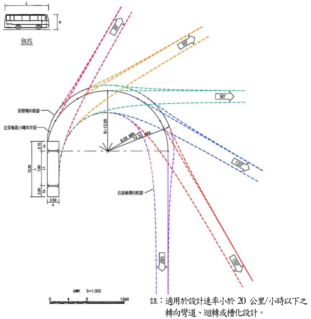
大客車最小轉向軌跡參考圖
