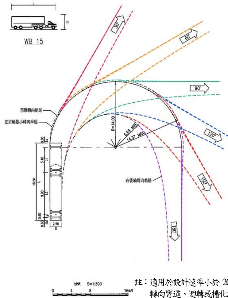
大型聯結車最小轉向軌跡參考圖
